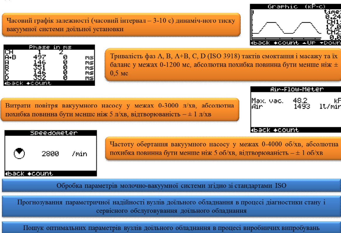
Рис. 2. Характеристика комплекту устаткування
