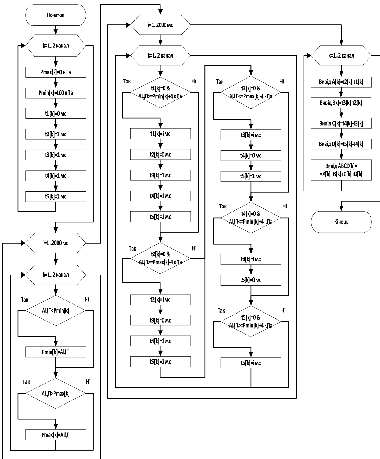
Рис. 7. Алгоритм визначення тривалості фаз A, B, C, D тактів смоктання і масажу та період пульсацій ABCD.
