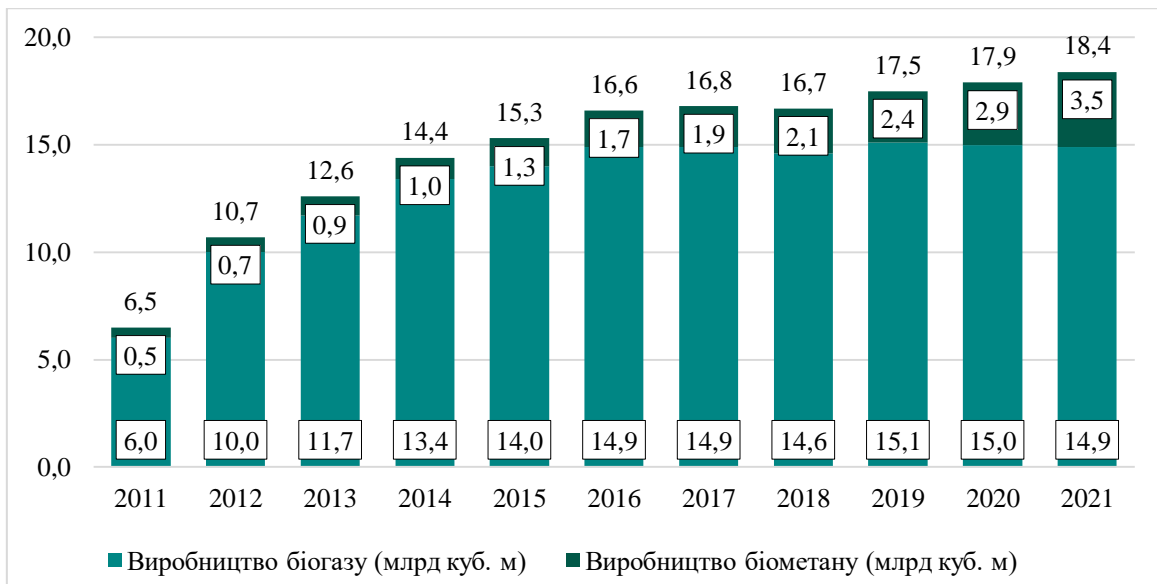
Рис. 4. Обсяги виробництва біогазу і біометану у країнах ЄС у 2021 р., млрд куб. м
