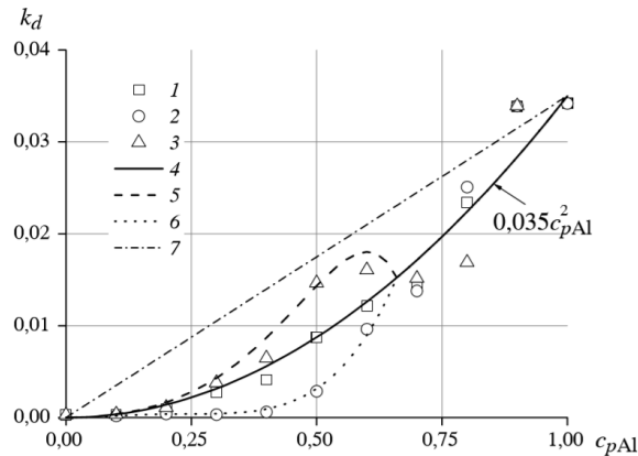
Рис. 12. Залежності коефіцієнтів напilenня суміші: 1 – алюмінію, 2 – міді, 3 – від концентрації алюмінію у вихідній суміші; 4 – параболічна апроксимація коефіцієнта напilenня суміші; 5 – апроксимація коефіцієнта напilenня міді; 6 – апроксимація коефіцієнта напilenня алюмінію; 7 – коефіцієнт напilenня суміші по лінійній теорії (коли компоненти не впливають один на одного)
