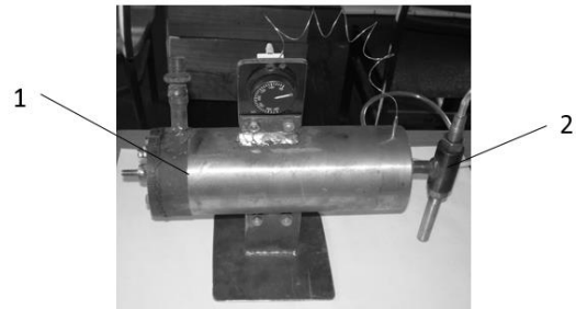
Рис. 4. Установка для холодного газодинамічного напилення (ХГДН) поверхневих шарів: 1 – нагрівач повітря, 2 – сопло.
