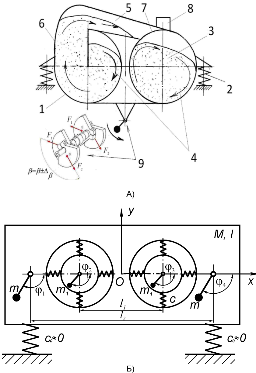
Рис. 2 а) просторово-циркуляційний рух завантаження у адаптивному вібротліні; б) тримасний вібраційний млин з чотирма вібробуджувачами
