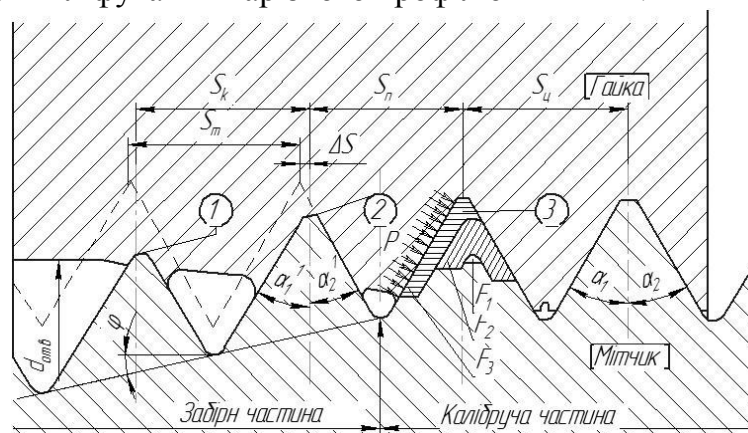
Рис. 1. Схема формування профілю різьби безстружечними мітчиками з кінчною схемою деформування
