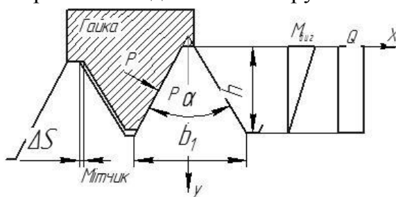
Рис. 2. Сили діючі на виток розташований в перехідній зоні
