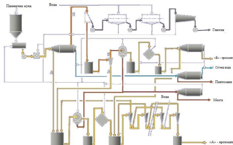
Рис. 2. Трьохфазний декантерний процес на прикладі компанії Alfa-Laval
