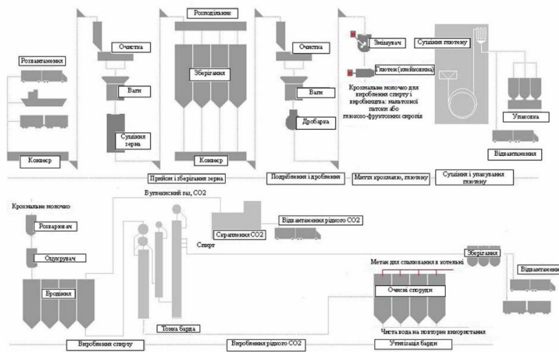
Рис. 1. Схема технологічного процесу глибокої переробки зерна
