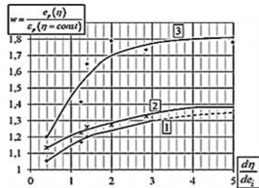
Рис. 5. Залежність коефіцієнта впливу історії деформування w від швидкості зміни показника напруженого стану
