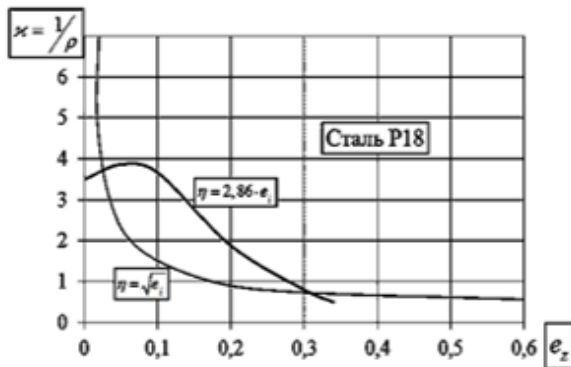
Рис. 7. Залежність кривизни траєкторії деформацій \chi від осьової деформації e_z циліндричних зразків, що піддаються крученню спільно з розтягом сталі P18 при \eta = \sqrt{e_i}, \eta = 2,86e_i
