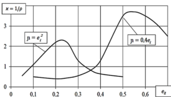
Рис. 8. Залежність кривизни траєкторії деформацій \chi від осьової деформації e_z циліндричних зразків, що піддаються крученню спільно з розтягом сталі P18 при \eta = e_i^2, \eta = 0,4e_i
