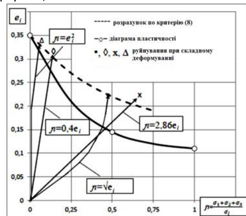
Рис. 9. Вплив історії деформування на пластичність сталі P18 [2]
